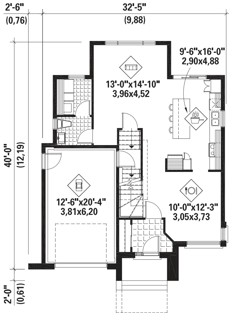
REZ-DE-CHAUSSÉE 818 PI. CA.
