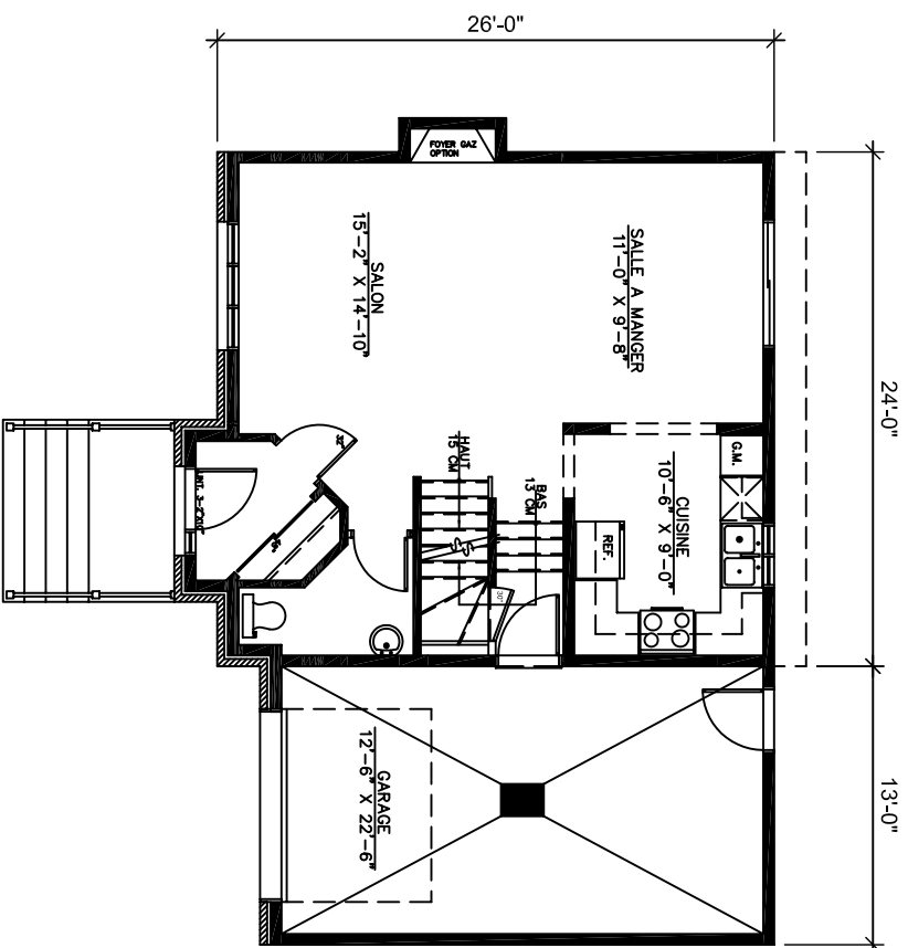
REZ-DE-CHAUSSEE 641 PL. CA.
