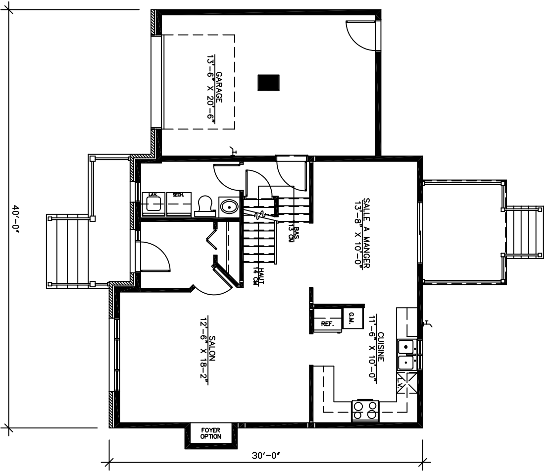
REZ-DE-CHAUSSEE 756.0 pi.ca.
