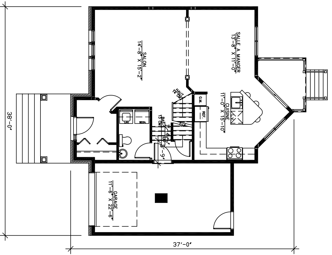
REZ-DE-CHAUSSÉE 798.0 pi.ca.
