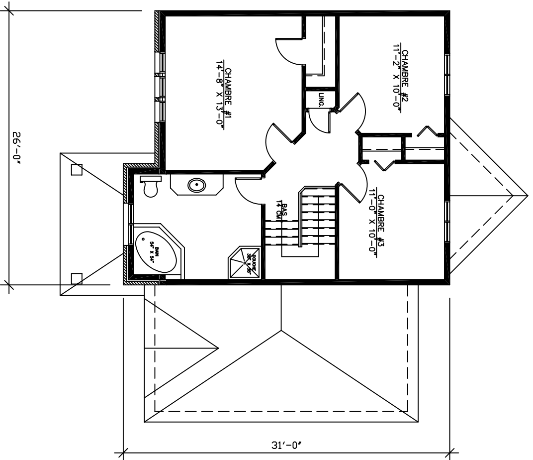
ÉTAGE 762.0 pi.ca.
