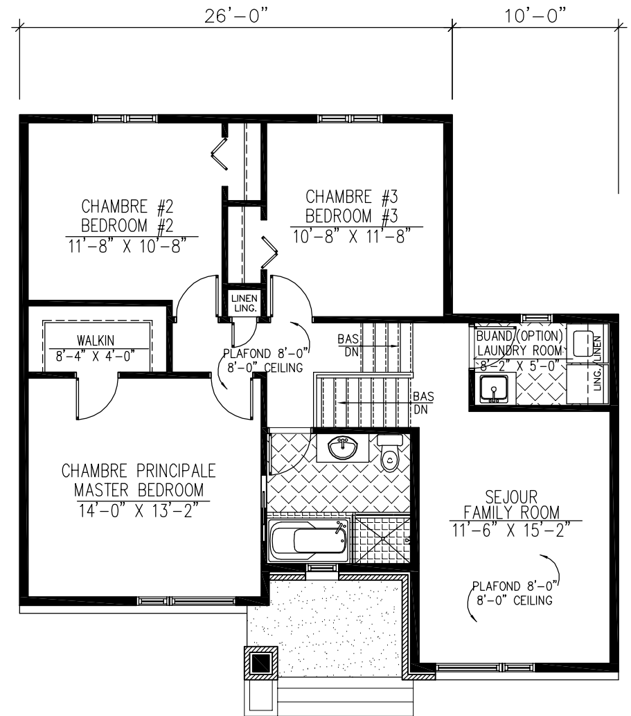
Étage/Upper Floor: 915 p.c.
