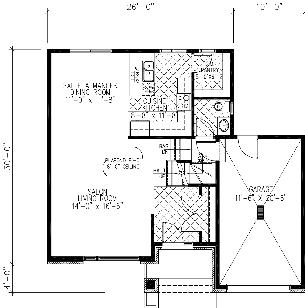
R-de-C/Main Floor: 728 p.c. Garage: 269 p.c.
